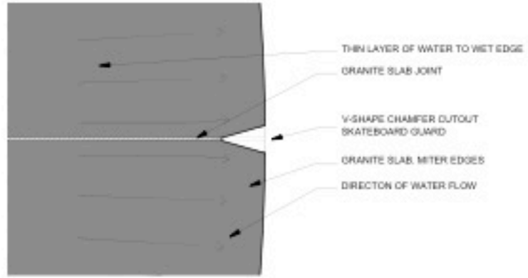
4 EDGE AND SKATEGUARD PLAN DETAIL SCALE: 6" = 1'-0"
