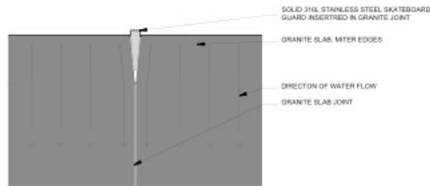
5 EDGE AND SKATEGUARD ELEVATION DETAIL SCALE: 1" = 1'-0"
