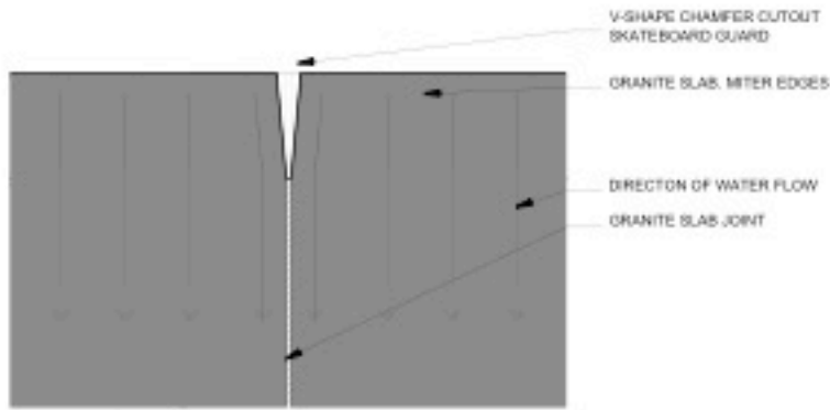
5 EDGE AND SKATEGUARD ELEVATION DETAIL SCALE: 6" = 1'-0"
