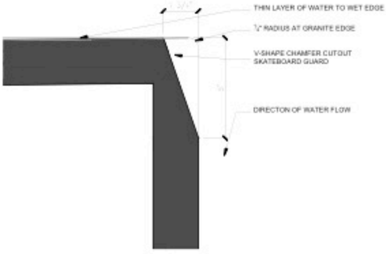
3 EDGE AND SKATEGUARD SECTION DETAIL SCALE: 6" = 1'-0"
